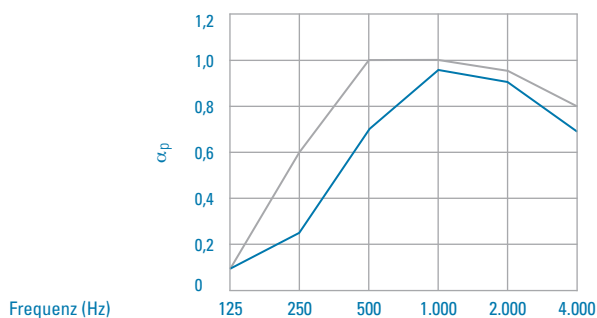
Schallabsorptionsgrad \alpha_p , pinta ARTWORK, nach DIN EN ISO 11854
