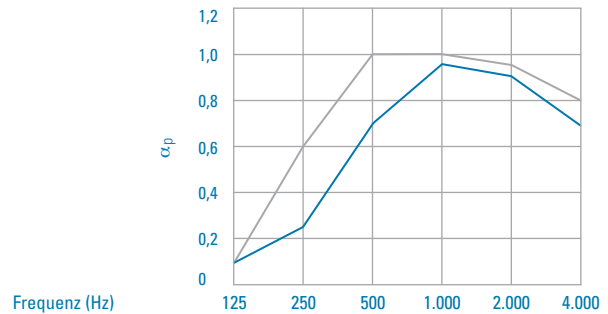
Schallabsorptionsgrad \alpha_p , pinta ARTWORK, nach DIN EN ISO 11654
