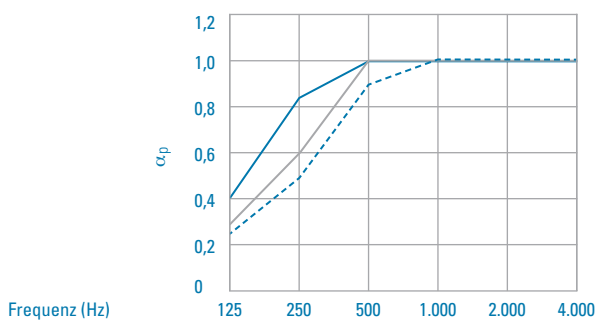
Schallabsorptionsgrad \alpha_p , pinta Absorber RONDO S, nach DIN EN ISO 11654
