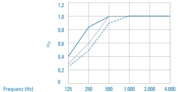
Schallabsorptionsgrad \alpha_p , pinta Absorber RONDO S, nach DIN EN ISO 11654
